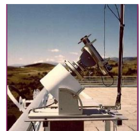
Pyréliomètre
